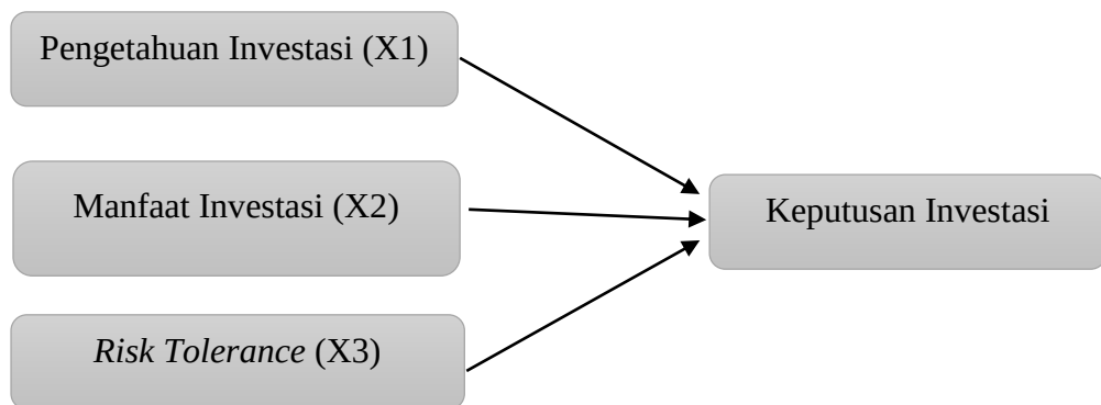
Gambar 3 Kerangka Pemikiran
